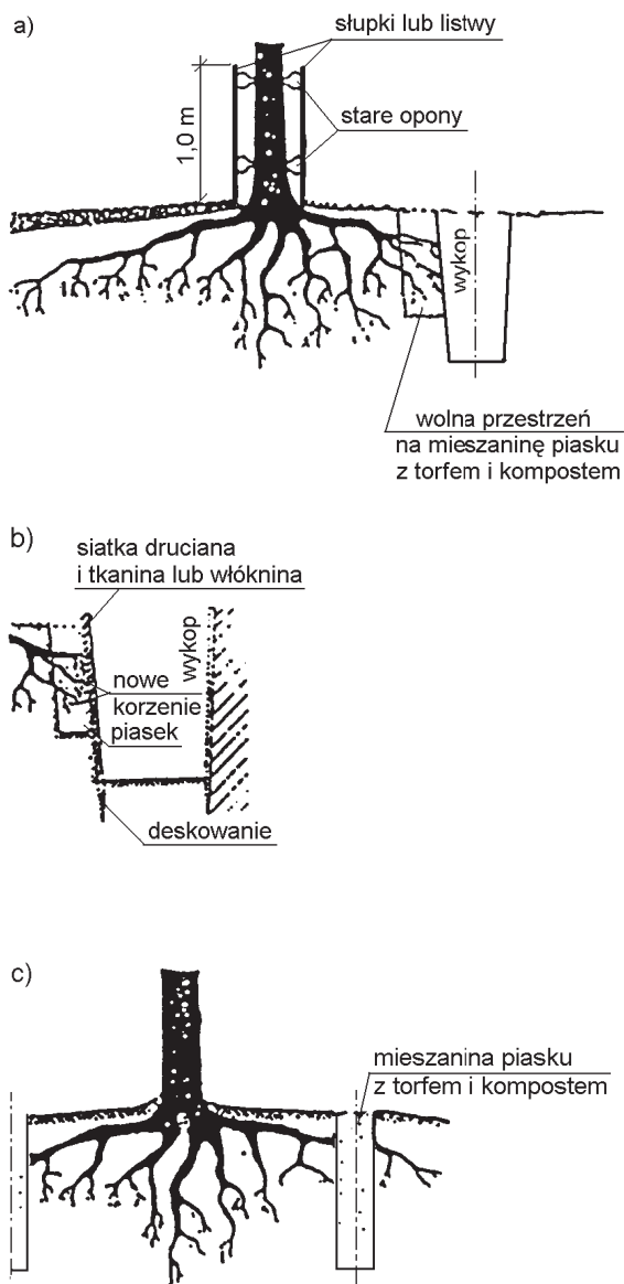
a) przekrój ogólny, b) szczegóły wykopu, c) wstępna faza zabezpieczenia, wykonywana najlepiej rok przed właściwym wykopem
